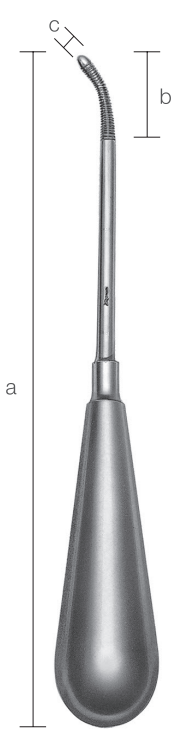
10222800 穿刺孔拡大やすり 木村・川上氏 a 180 b 25 c 4
