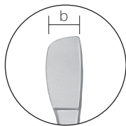
10223300 齒齦切開刀 田所氏 全長 140 a 17 b 8.1
