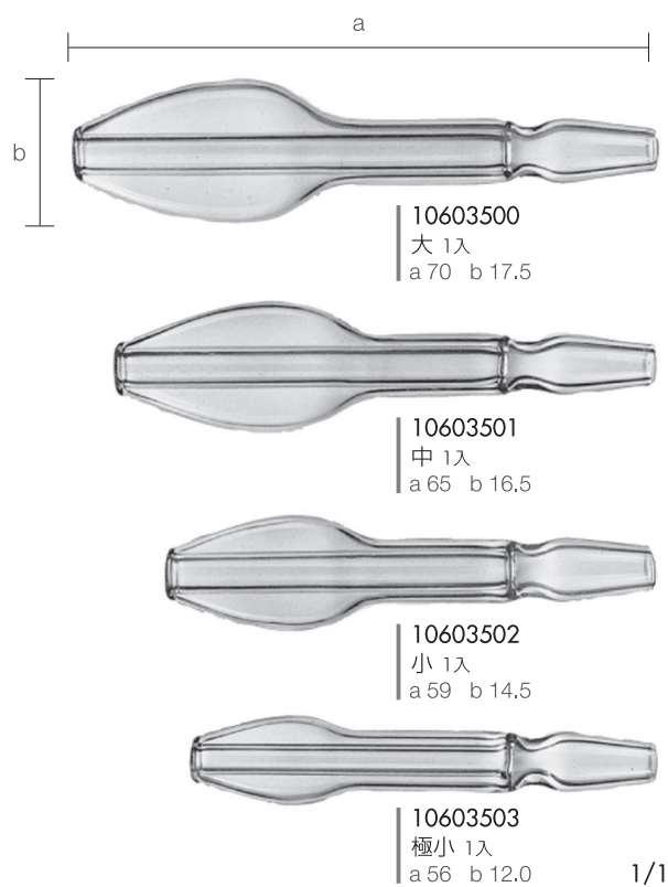
吸引用オリフ N-40
