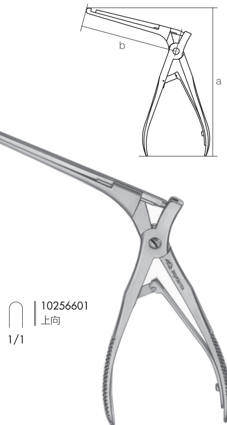
篩骨蝶形洞彫骨器 足川氏 細型 a 217 b 170 c 5.7 d 5
