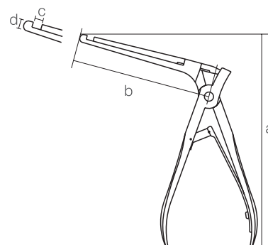
耳小骨剪刀 後藤敏郎氏 全長 105 a 25
