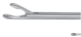
10146400 極小鋭匙鉗子 直 a 110 b 75
