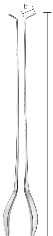
* 10214700 上顎洞消息子 キリアン氏 左右 11mm a 205 b 11
