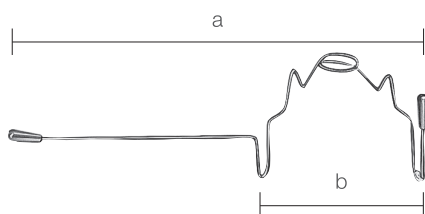
10200700 針金鼻鏡 左 a 95 b 40
