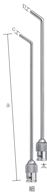
* 10306200 扁桃窩洗浄器 野坂氏 (5cc) (先 太・細 各1本付) a 100 b 2.4 c 1.7
