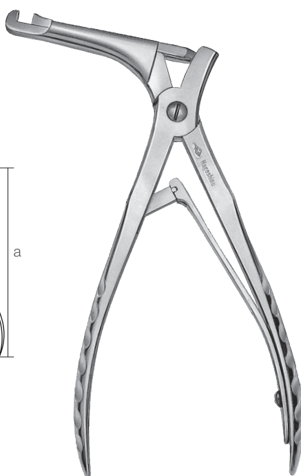
10228500 骨止血器 スタンツェー型 岩田氏 a 153 b 67 c 5.3 d 8.6
