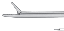
10148200 超極小麦粒鉗子 直 a 115 b 75
