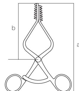
10143373 開創器 帝京大型 C 爪長/足長 梨地 a 175 b 110 c 27 d 16
