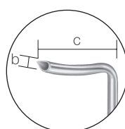
10215201 鋭先／長(17mm) b 2.1 c 17
