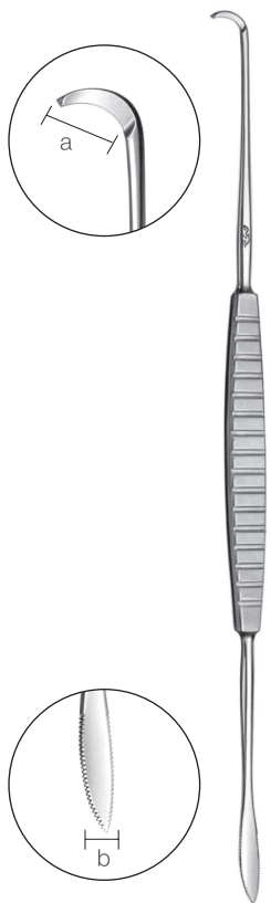
10305500 扁桃摘出刀 笹木氏 全長 240 a 12 b 7
