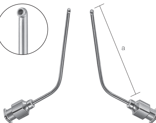
* 10123900 鼓室洗浄管 ハルトマン氏 左右 a 62
