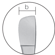
10223200 齒齦切開刀 石橋氏 全長 155 a 16 b 8.9
